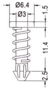
P.C.B Ø3.0
