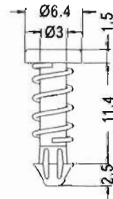
P.C.B Ø3.0
