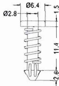
P.C.B Ø3.0
