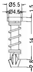
P.C.B Ø3.0
